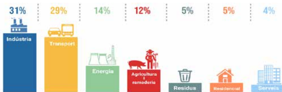
Distribució de les emissions de CO2 per activitats (2018) - Font: Oficina del Canvi Climàtic
